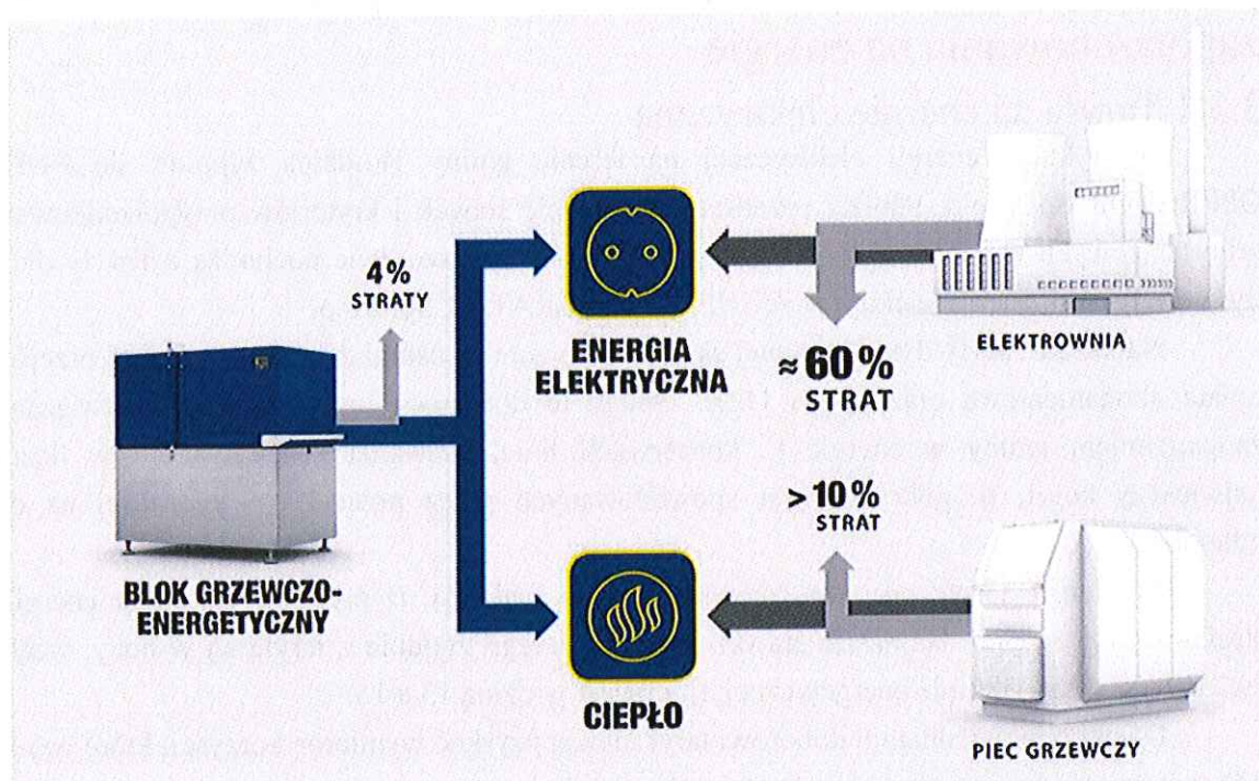
Rysunek 6 Schemat systemu kogeneracji
