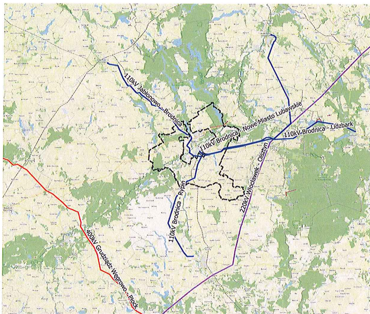
Mapa 3 Zasilenie w wysokie i najwyższe napięcia
